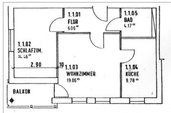
Wohnbeispiel (Grundriss)
