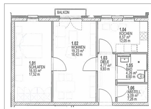
Wohnbeispiel (Grundriss)
