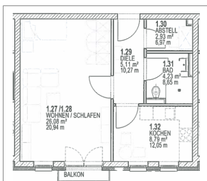
Wohnbeispiel (Grundriss)
