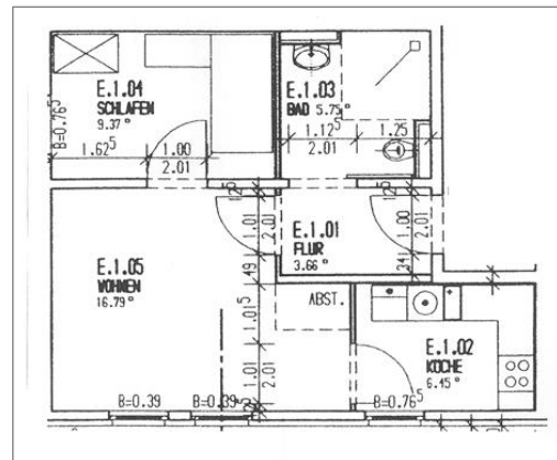
Wohnbeispiel (Grundriss)
