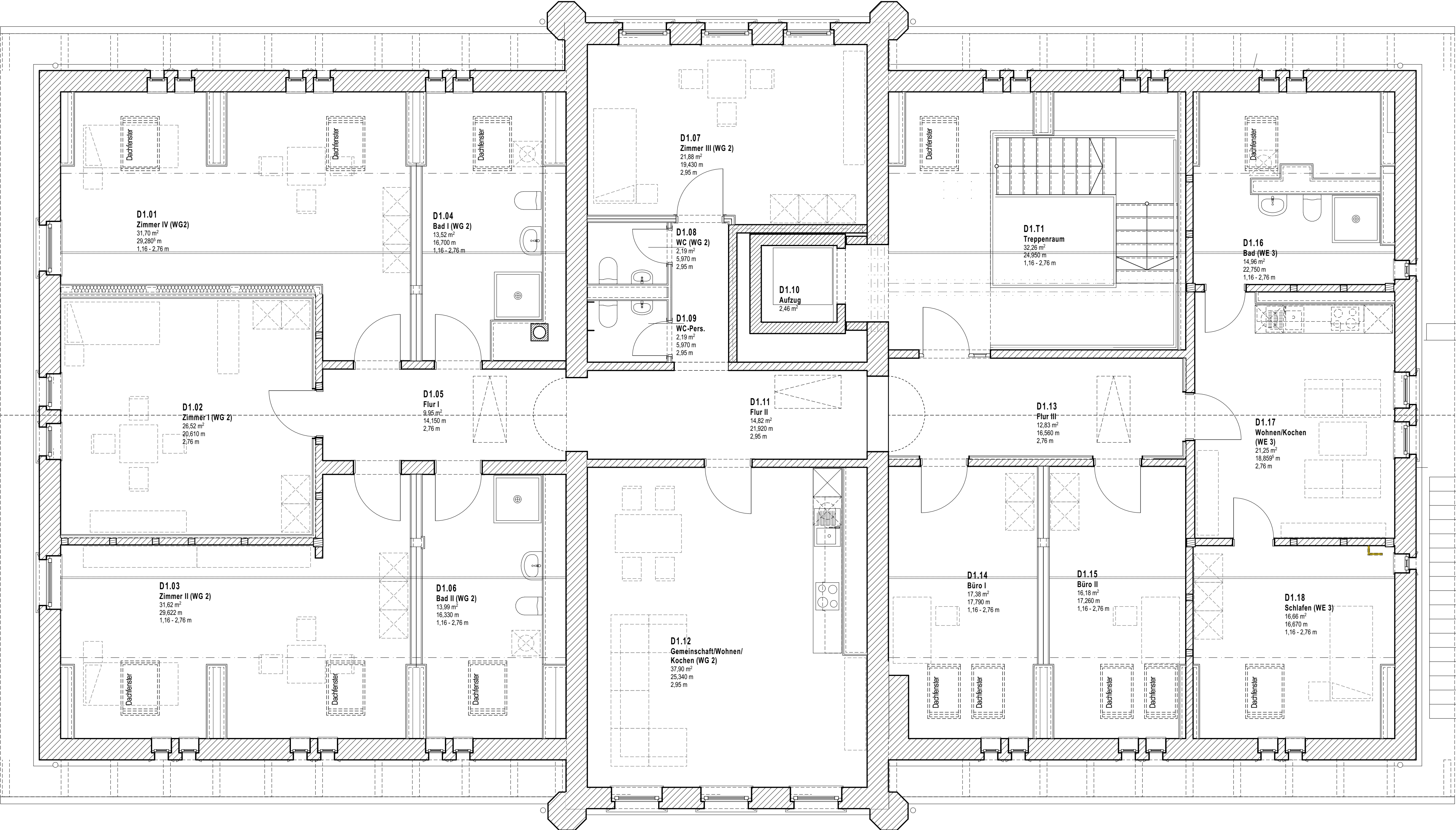
Grundriss 1. Dachgeschoss M = 1 : 50
