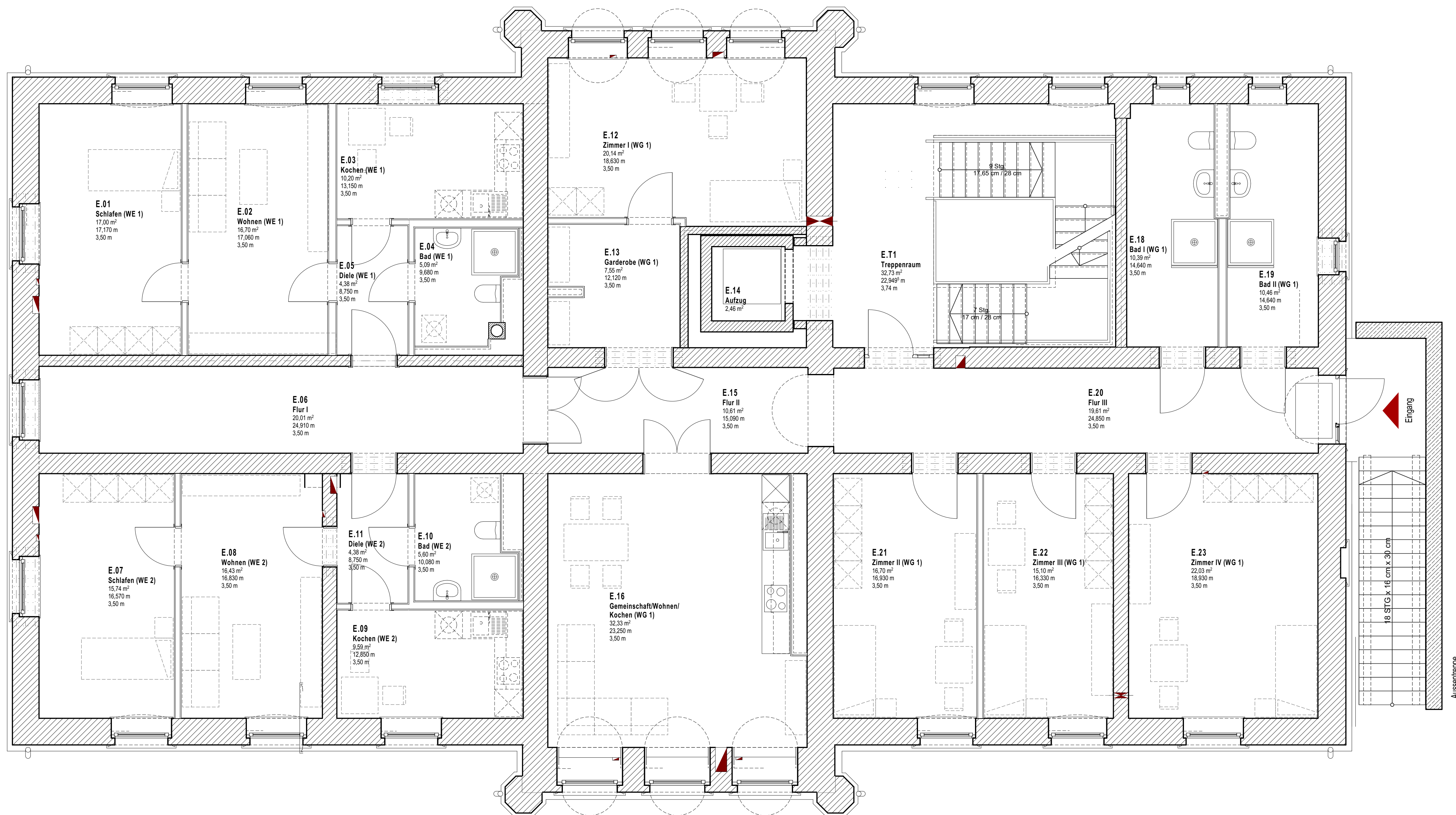
Grundriss Erdgeschoss M = 1 : 50
