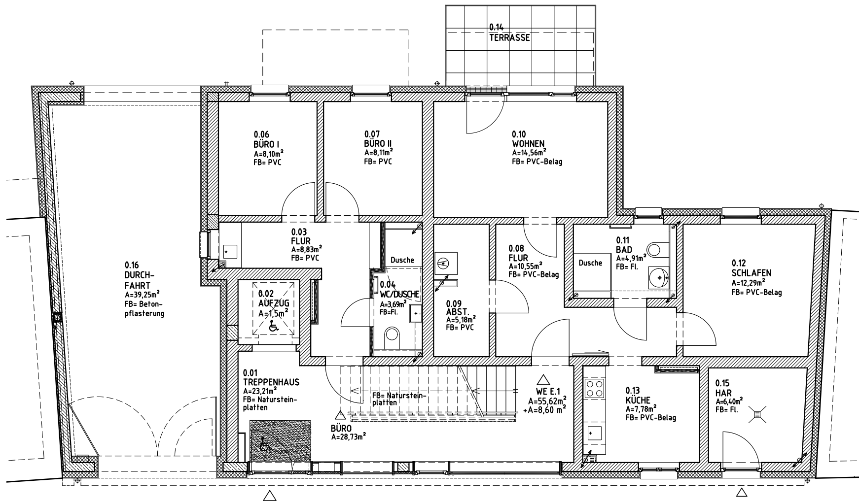
ERDGESCHOSS
